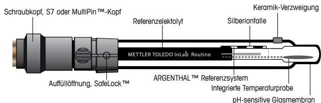
Bild 11. Typische pH-Kombinationselektrode mit einem inneren pH-Sensor und einem äußeren Referenzelement.
