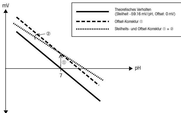
Bild 13. Korrelation zwischen dem von der pH-Elektrode gemessenen mV-Wert und dem pH-Wert der Probe. Die abgebildeten Kurven gelten für das theoretische Verhalten, für Verhalten mit Offset-Kompensation und für Verhalten mit Steilheits- und Offset-Kompensation.
