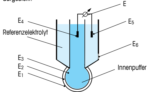
Bild 24. Die verschiedenen Potentialquellen einer Kombinationselektrode
